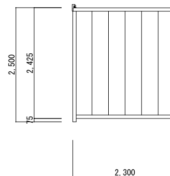
D面 立面図 S=1/60
