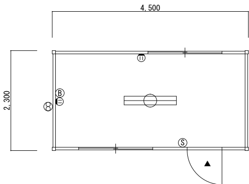
平面図 S=1/60
