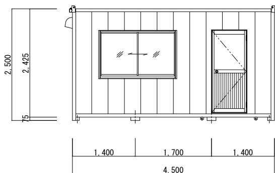
A面 立面図 S=1/60
