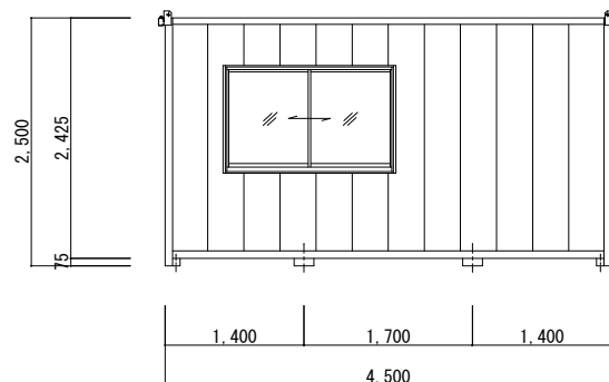
C面 立面図 S=1/60
