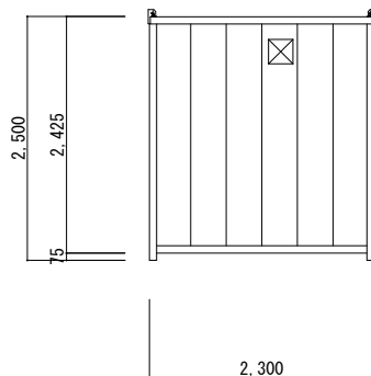
B面 立面図 S=1/60
