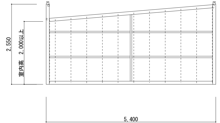
B面 立面図 S=1/60
