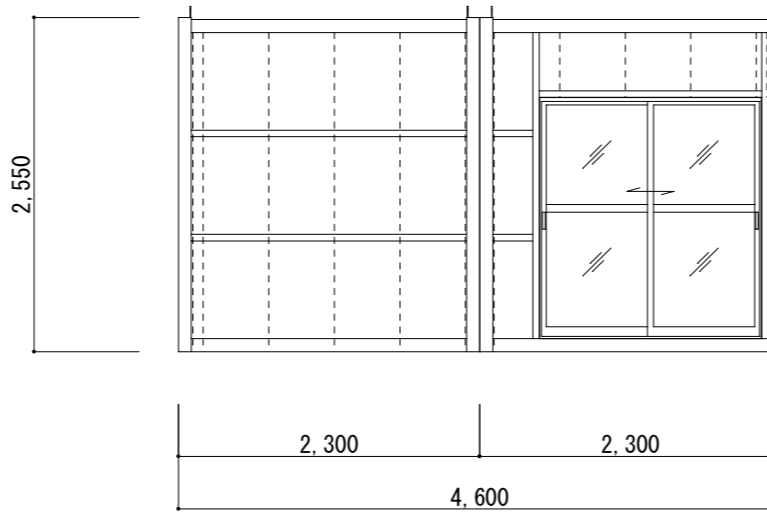
A面 立面図 S=1/60
