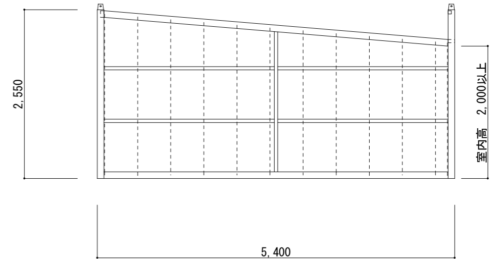
D面 立面図 S=1/60
