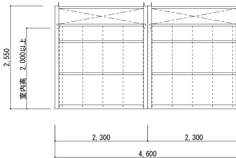
C面 立面図 S=1/60
